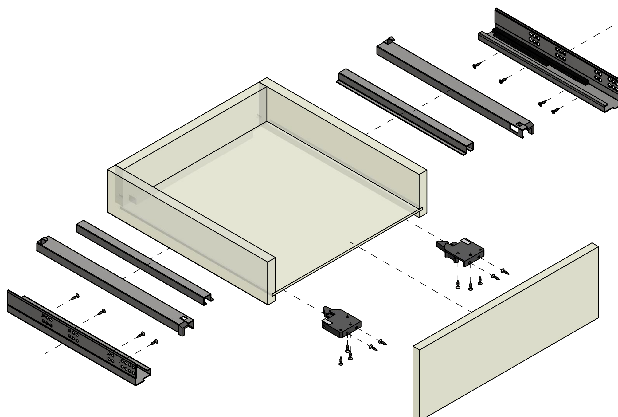
Montaż prowadnic do szuflady i korpusu
